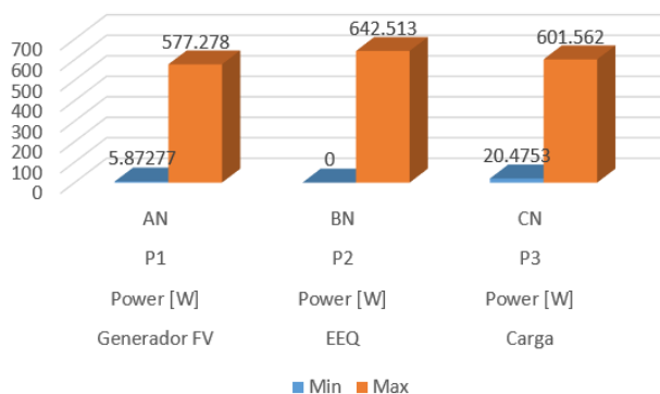
Figura 6. Potencia genrada y consumida por el sistema.
