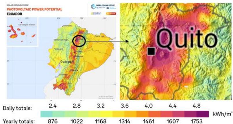
Figura 3. Potencial de generación fotovoltaica. Histórico 1999-2015 Fuente: Solargis, 2017
