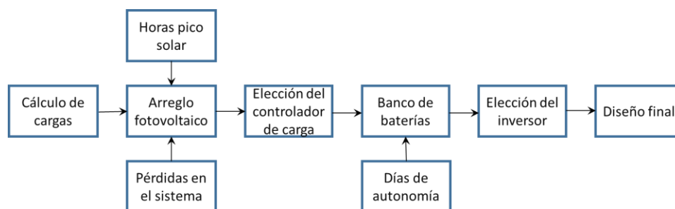
Figura1. Proceso de diseño de sistema de generación fotovoltaica.
