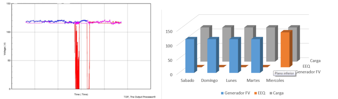
Figura 5. Voltajes del sistema fotovoltaico. a) Equipo de medición. b) Datos tabulados
