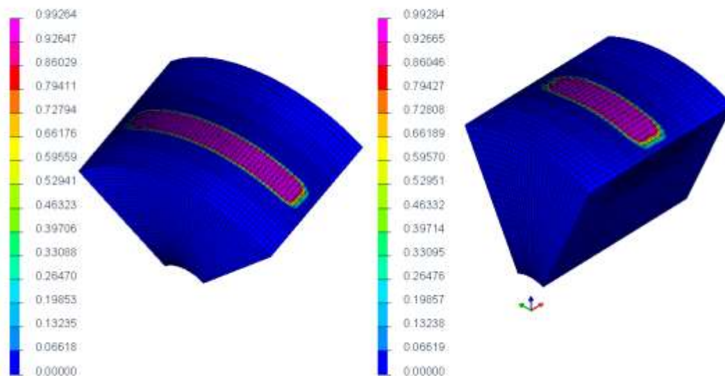
Gráfico 2. Caso práctico, geometrías de 50^\circ y 90^\circ de sección, dos pasadas de láser en cada pieza. En colores se indica el porcentaje de concentración de martensita.
