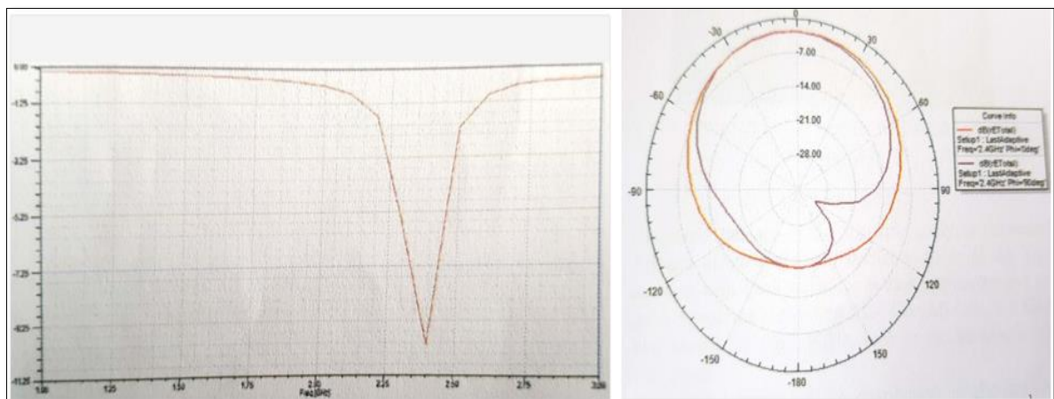
Figura 4. Antena Tribanda (Yagui) resonancia de frecuencias y patrón de radiación, Frecuencia de 2.4 GHz
