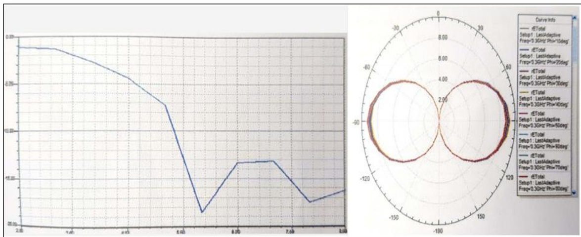
Figura 6. Antena Tribanda (Yagui) resonancia de frecuencias y patrón de radiación, Frecuencia de 5.5 GHz
