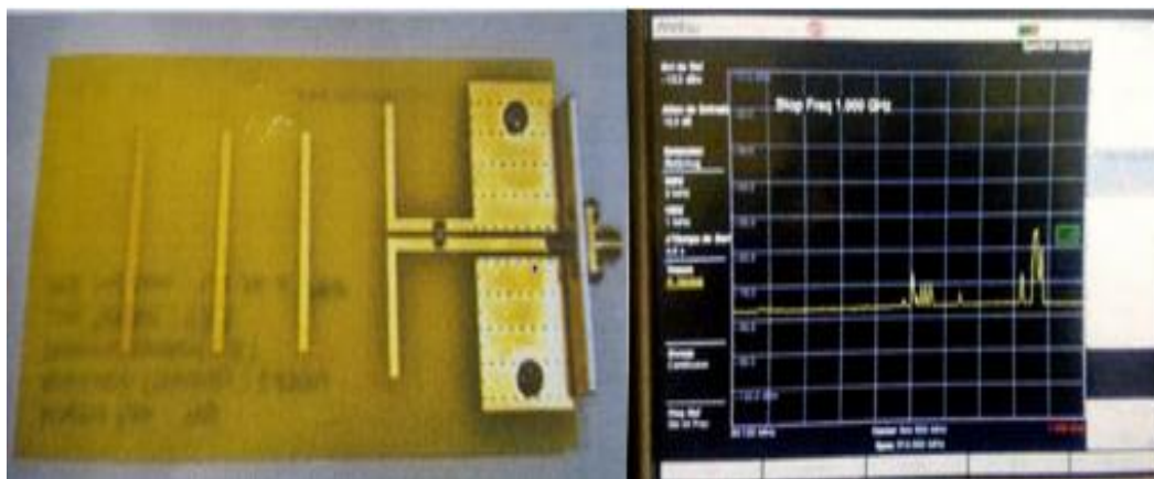
Figura 9. Antena Patch Diseño y recepción de señal
