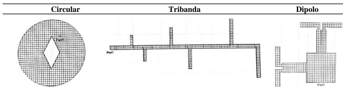
Figura 1. Diseño de antenas en Ansoft Designer
